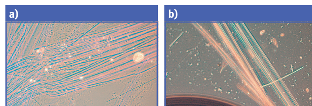
Figura 2: Fasci di crisotilo (a) e crocidolite (b) presente in un tramezzo in cemento-amianto osservato in microscopia ottica in contrasto di fase.
